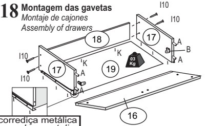
corredeira metálica corredera metálica metallic slide
